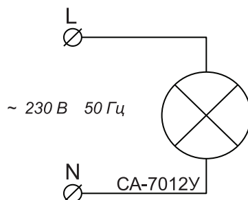
Рисунок 3. Схема подключения светильника CA-7012У
